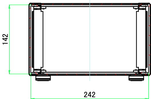
A-A ( 1 : 4.5 )
