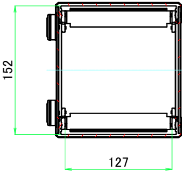
B-B ( 1 : 4.5 )
